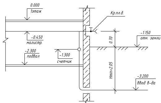
Рисунок 3 - Схема к определению отметок трубопроводов на вводе
