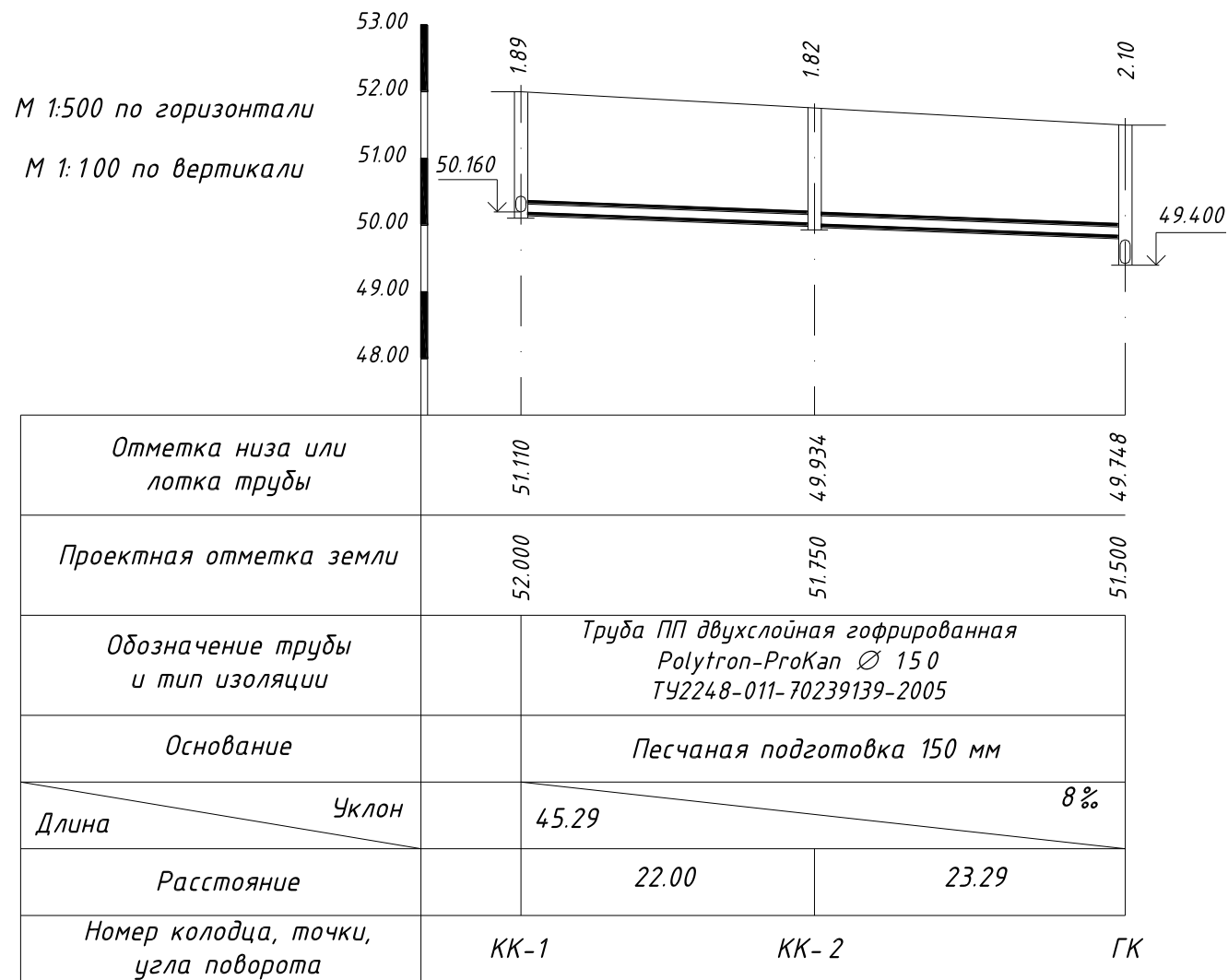
Рисунок 10 - Пример. Профиль внутриквартальной сети канализации
