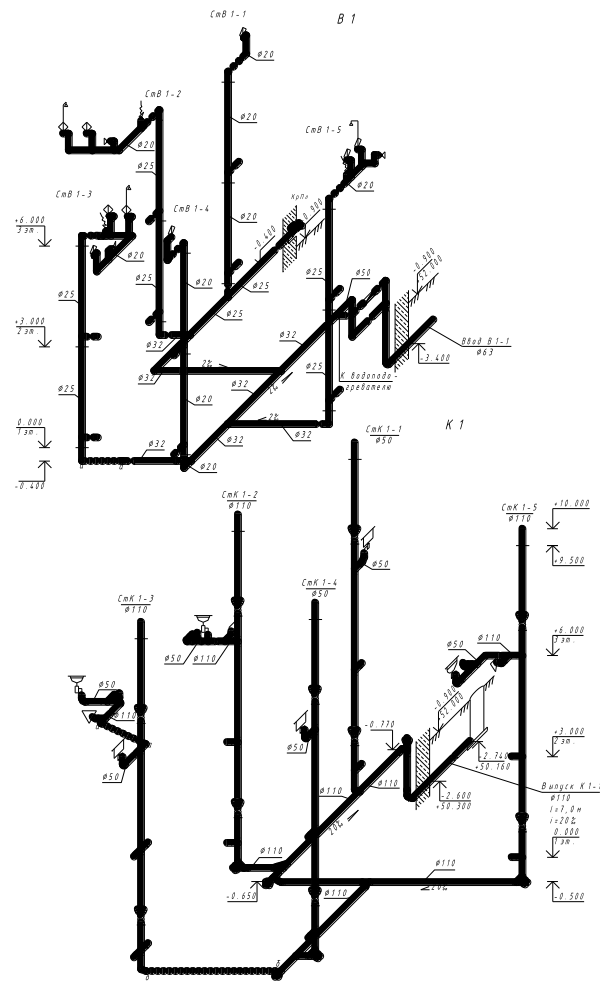
Рисунок 6 - Пример. Аксонометрические схемы водопровода и канализации
