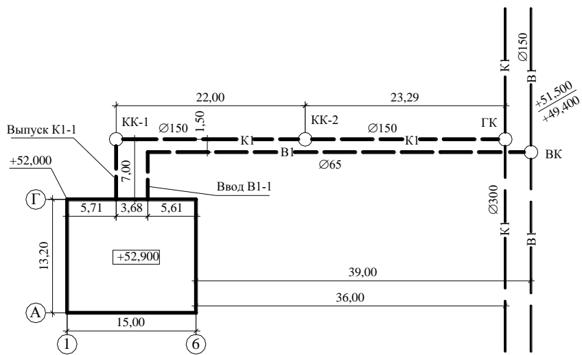
Рисунок 9 - Пример. Генплан участка
