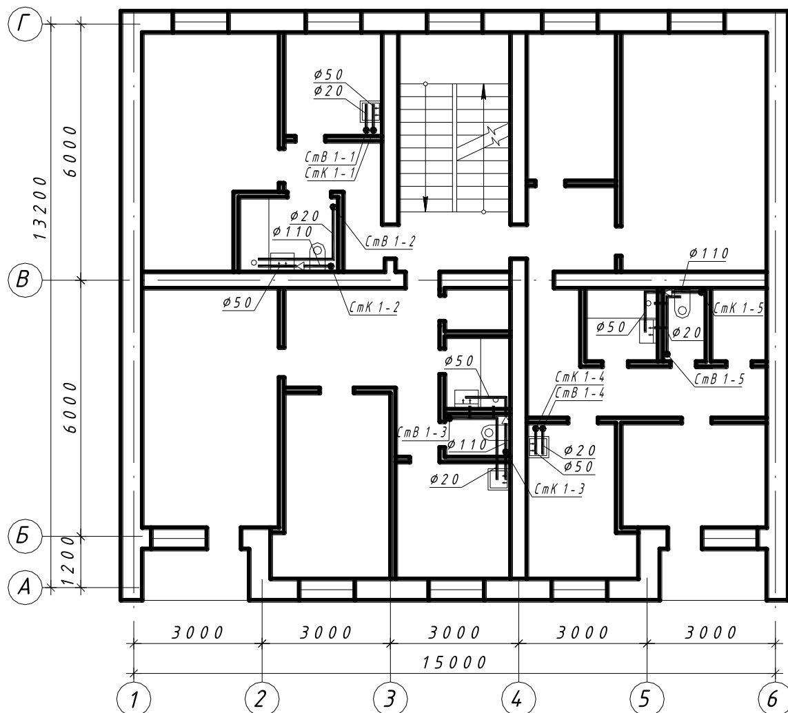
Рисунок 4 - Пример. План типового этажа
