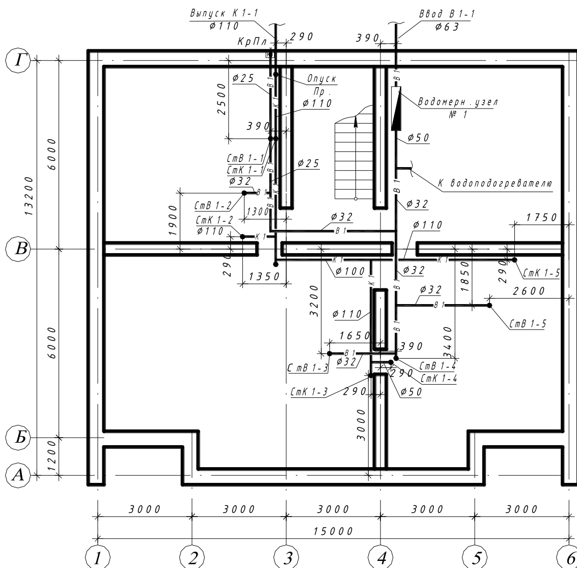
Рисунок 5 - Пример. План подвала
